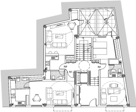
PLANTA BAJA
